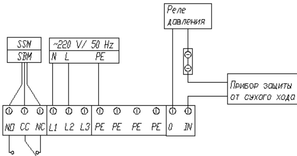
Рис.3 Схема электрических соединений.
